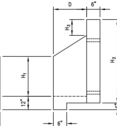
SIDE ELEV.
