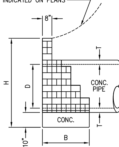
END ELEVATION
